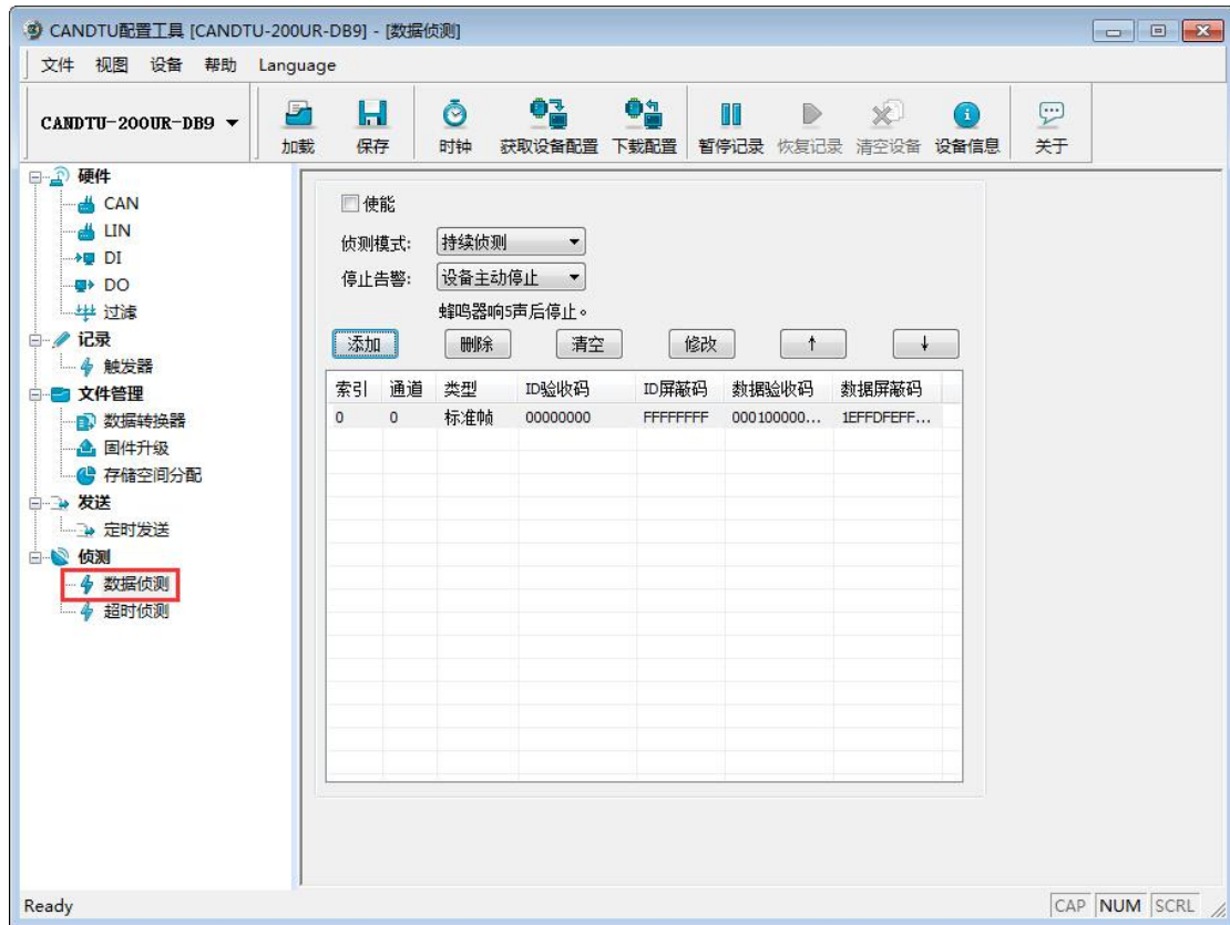
图 4.29 数据侦测选项卡
