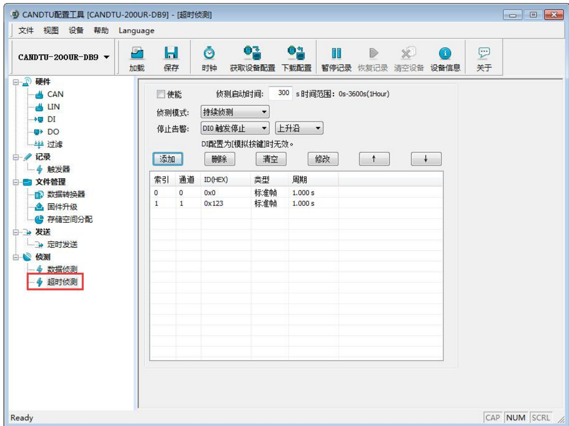
图 4.33 超时侦测选项卡
