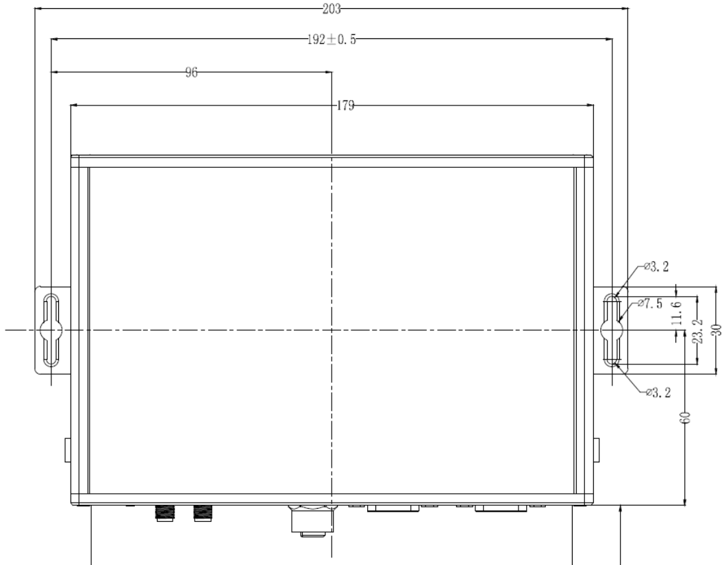
图 2.2 安装方式一
