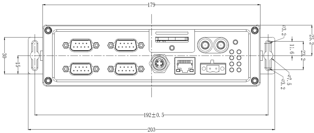
图 2.3 安装方式二
