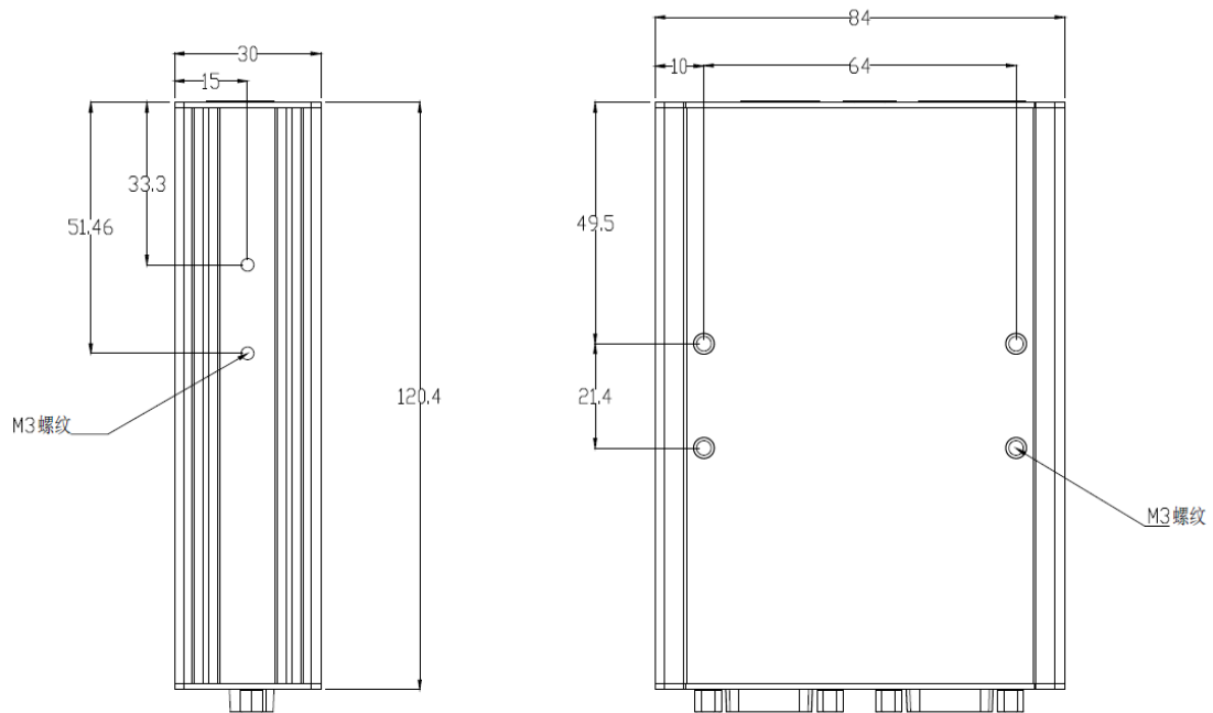
图 3.1 主机尺寸图
