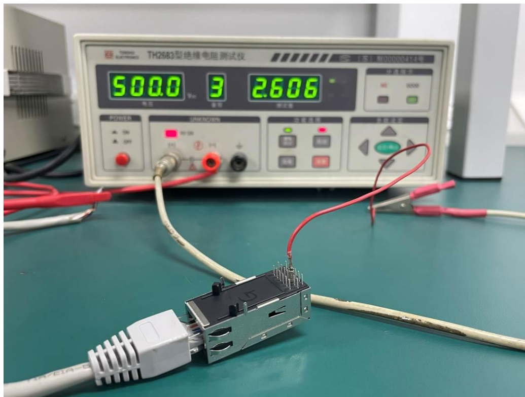
图 2 绝缘电阻试验
