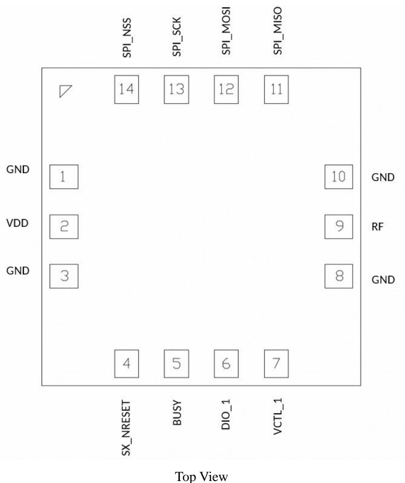
图 1.1 引脚分布图
