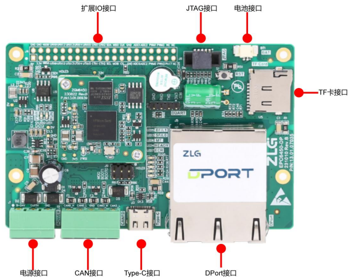
图 2.1 EPC6450-DP 评估板 A 面
