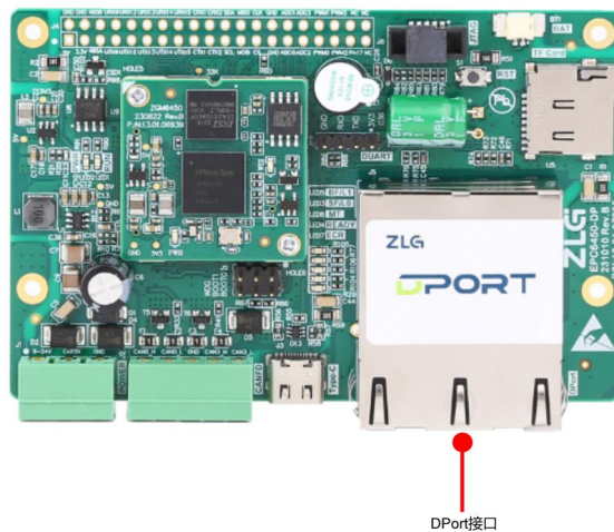
图 3.5 DPort 接口图
