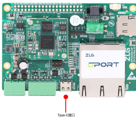
图 3.6 Type-C 接口图
