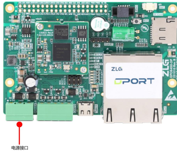
图 3.1 电源接口图
