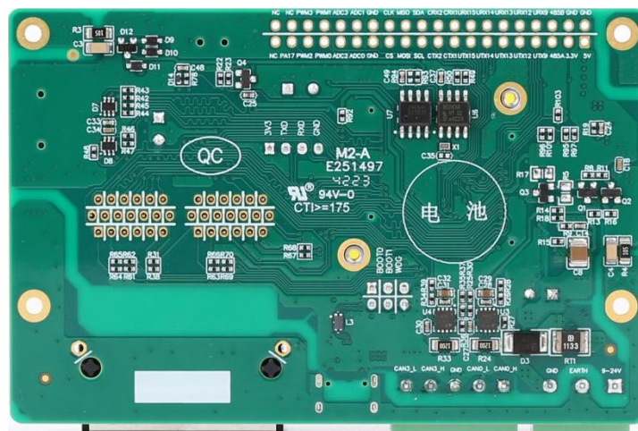
图 2.2 EPC6450-DP 评估板 B 面
