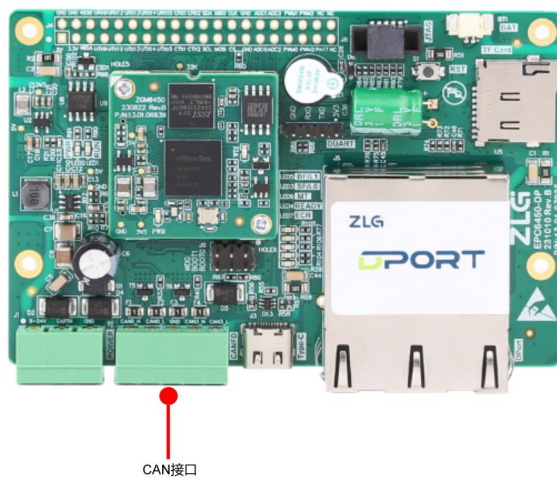
图 3.4 CAN 接口图
