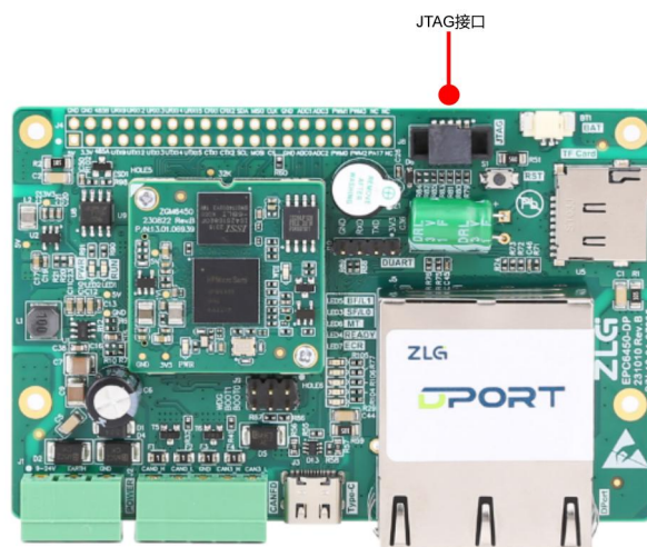
图 3.2 JTAG 接口图
