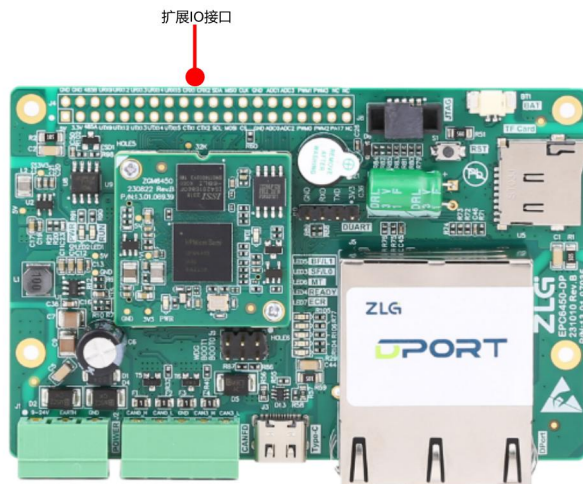
图 3.10 扩展 IO 接口图
