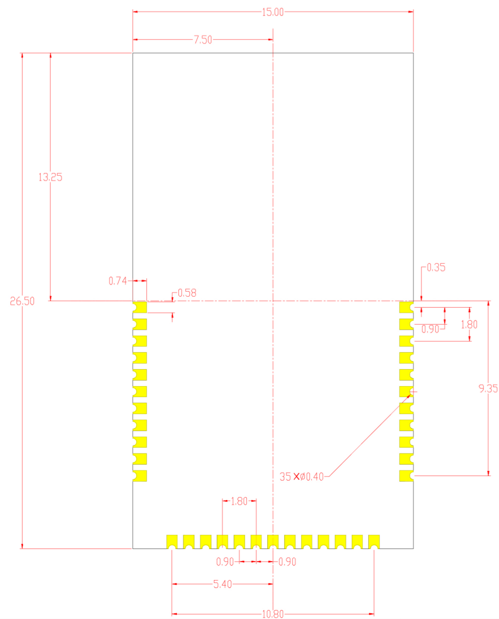
BOTTOM视图
