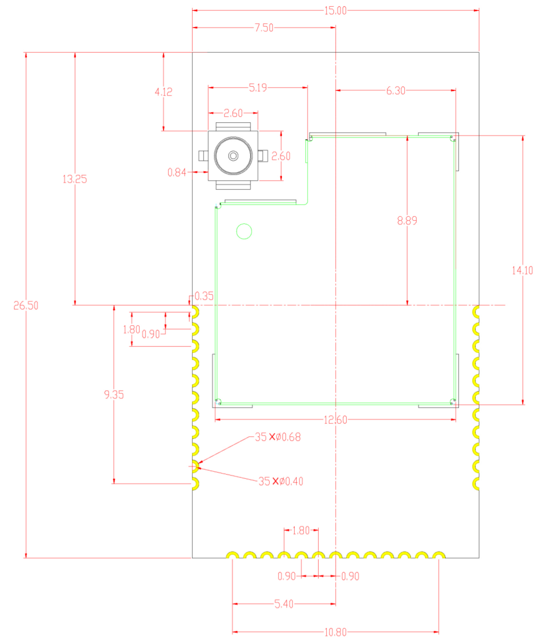
FRONT视图
