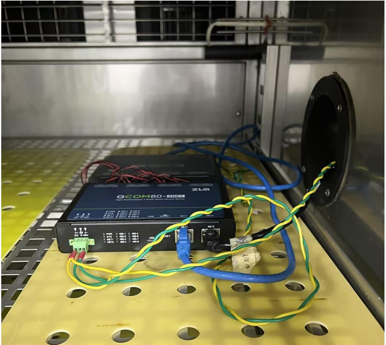
图 1 样机环境适应性试验
