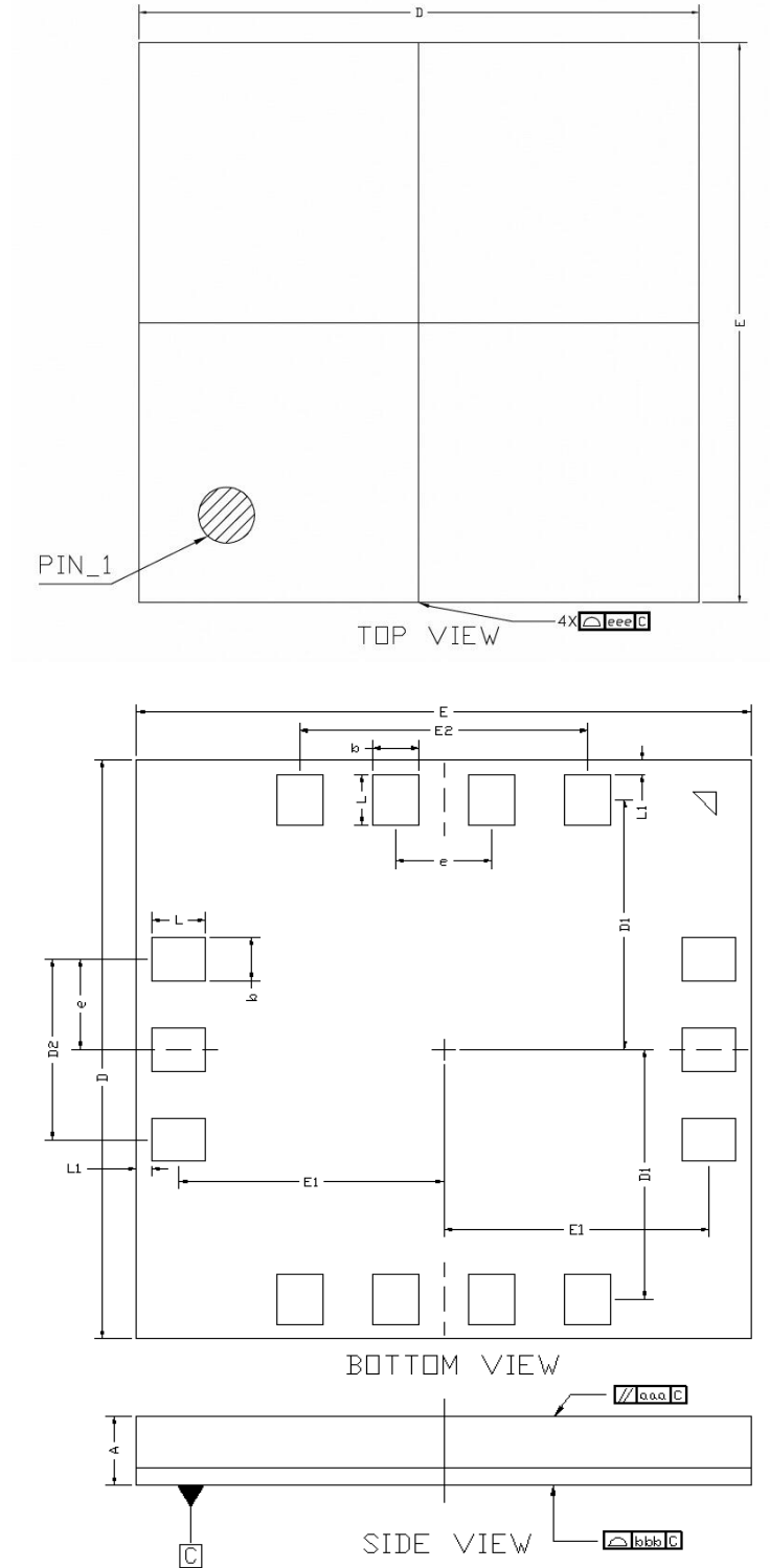
图 3.1 芯片尺寸
